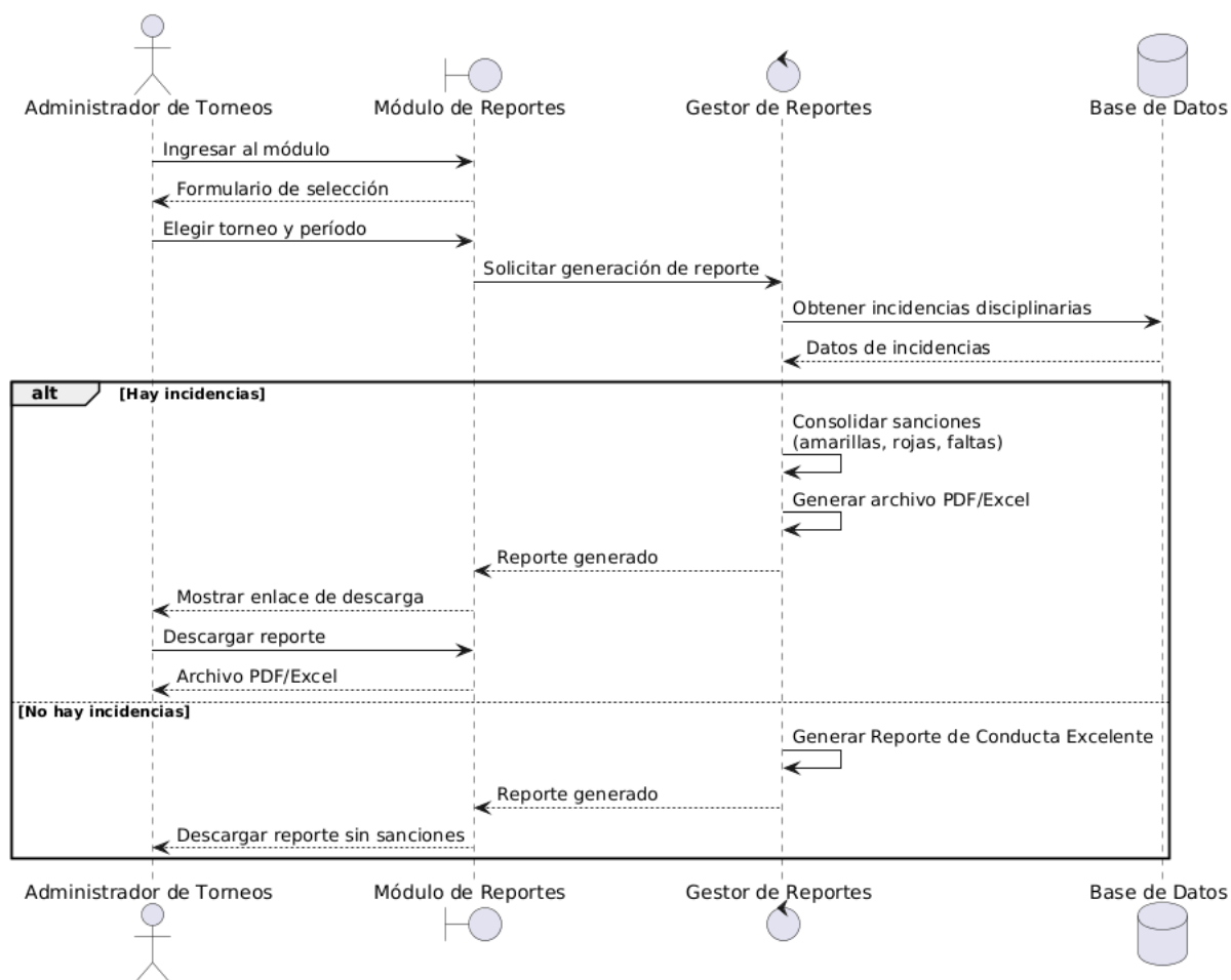
Ilustración 31 Diagrama de secuencia UC-06
